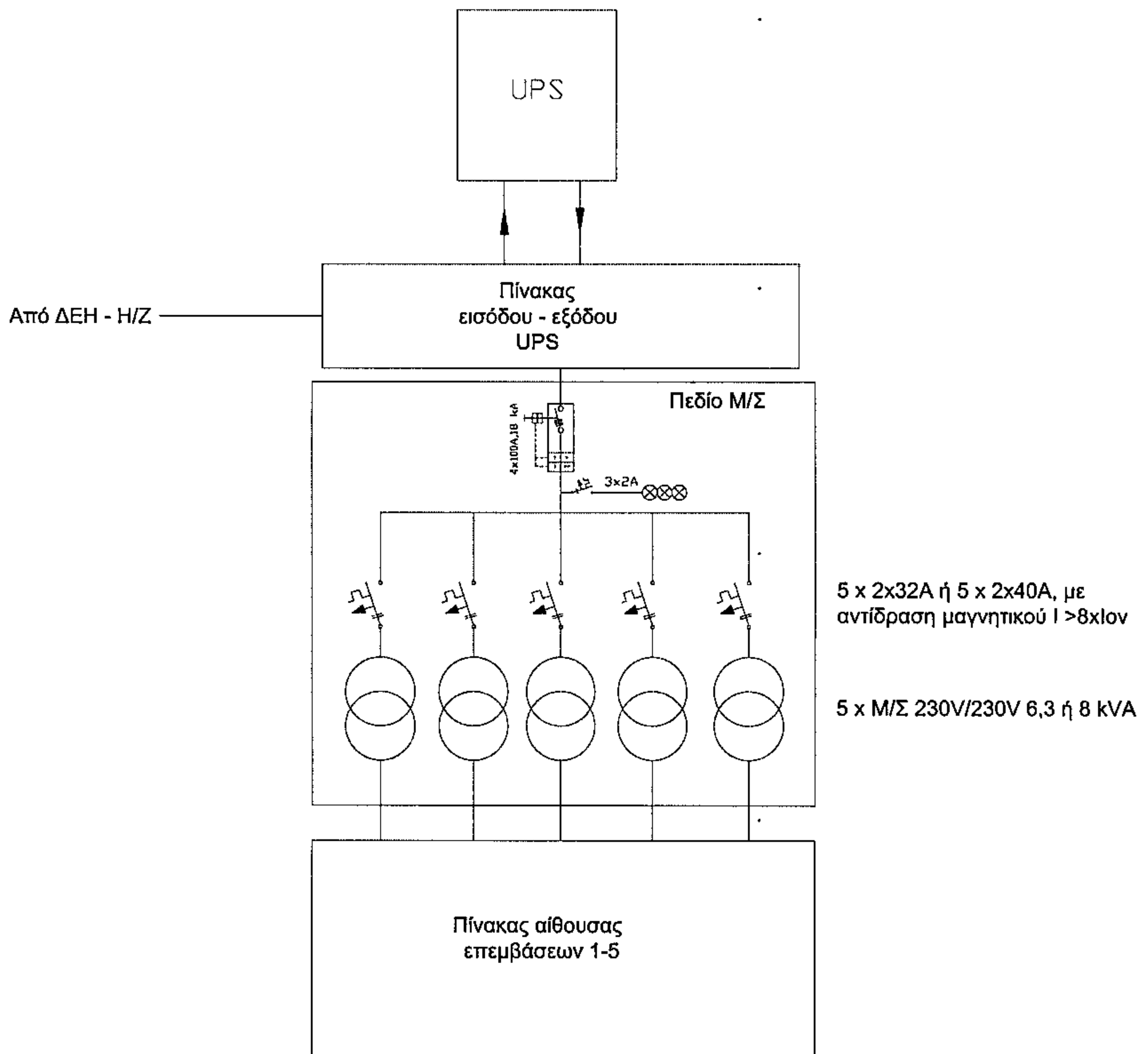
Διάγραμμα διανομής ισχύος από UPS σε πίνακα αίθουσας επεμβάσεων ΛΥΣΗ 2
