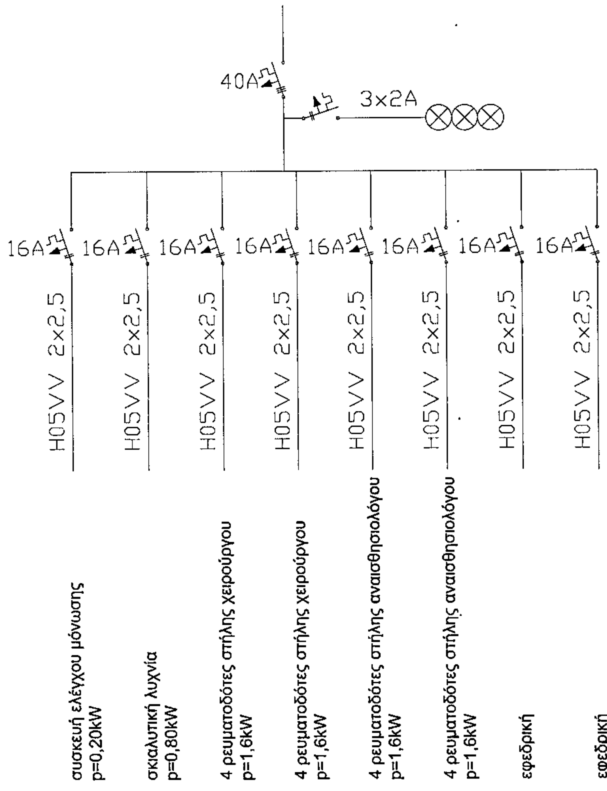
Ηλεκτρικός Πίνακας από ΔΕΗ - ΗΖ - UPS αίθουσας επεμβάσεων
